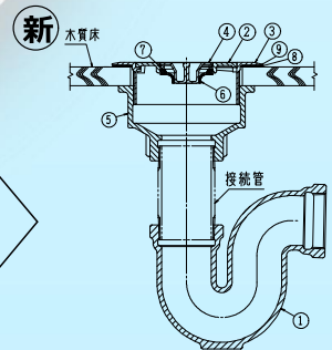
構成部品表
